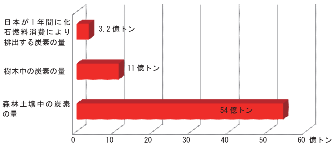
日本の森林内に蓄えられている炭素量の計算値 (太田誠一, 1998)
